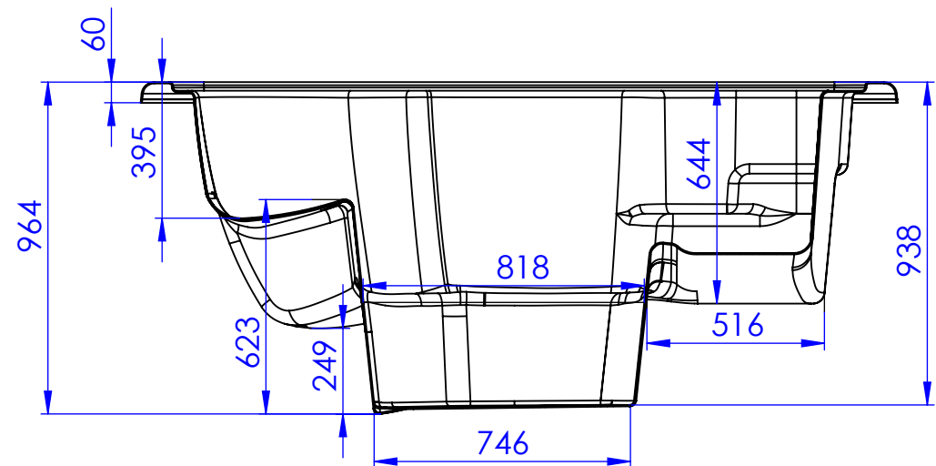
PJŪVIS A-A
